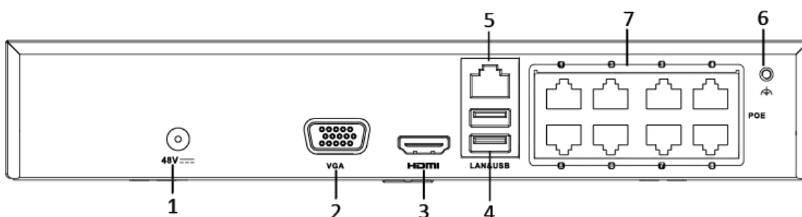
Abbildung 1-6 HWN-2100MH-P Rückpanel
